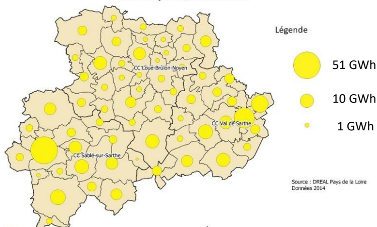
Potentiel de production d'électricité issue du solaire photovoltaïque sur le Pays Vallée de la Sarthe
